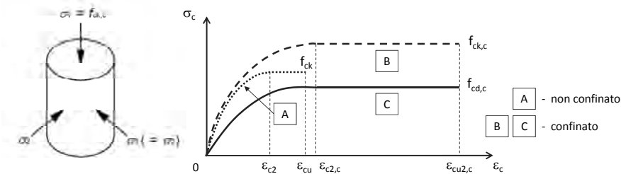
Fig. 4.1.2 - Modelli σ-ε per il calcestruzzo confinato
