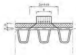
Fig. 5.1.3.b - Diffusione dei carichi concentrati negli impalcati a piastra ortotropa
